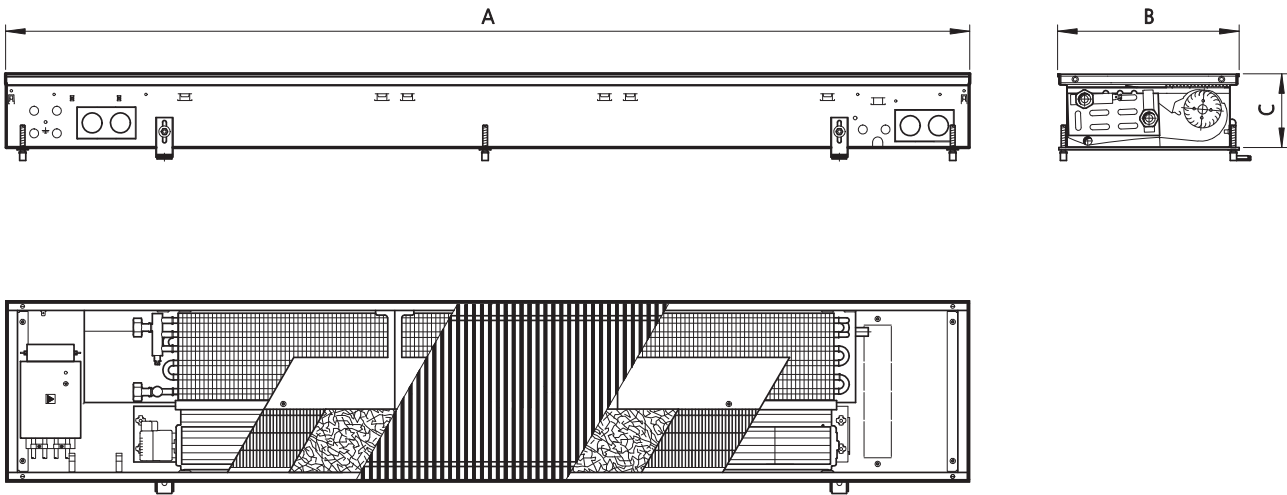
Технический чертёж (Размеры в мм)
